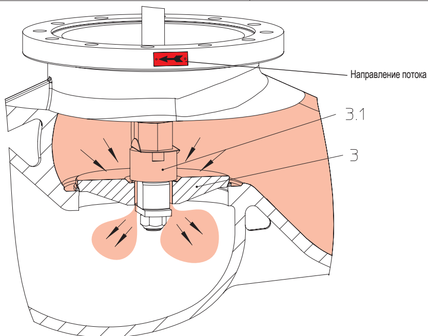
Дросселирующий затвор с конической посадочной поверхностью (макс. доп. \Delta P см. приложение: Характеристики расхода)
