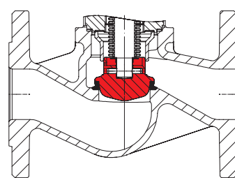
Дросселирующий затвор с мягким уплотнением из PTFE + 25% графита, максимальная рабочая температура 200°C (макс. доп. \Delta P см. приложение: Характеристики расхода)
