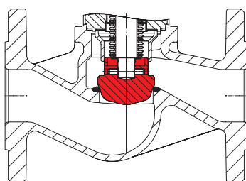
Дросселирующий затвор с конической посадочной поверхностью (макс. доп. \Delta P см. приложение: Характеристики расхода)
